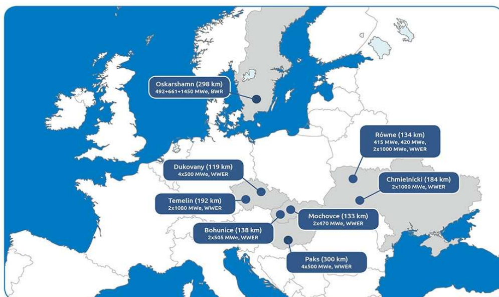
Lokalizacja elektrowni jądrowych w odległości ok. 300 km od granic Polski (źródło: PAA)
